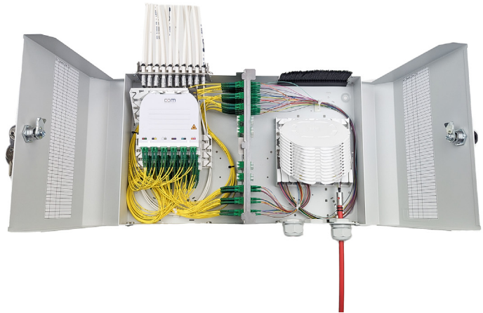
CCM Open Access Gehäuse (Abbildung ähnlich)
