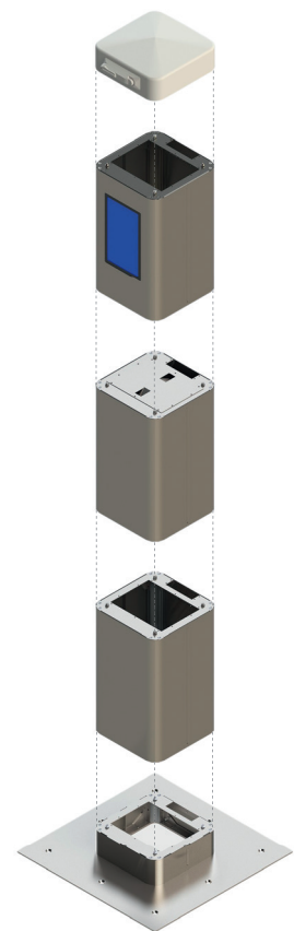
Modularer Aufbau CCM FiberSTELE
