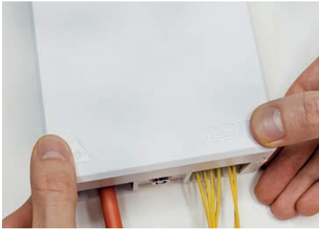
8B Deckel mit leichtem Druck oberhalb der seitlichen Druckpunkte bis zum Einrasten im Gehäuseboden verschließen.
